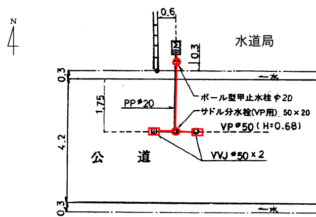
平面図 本管深度 h=0.68
