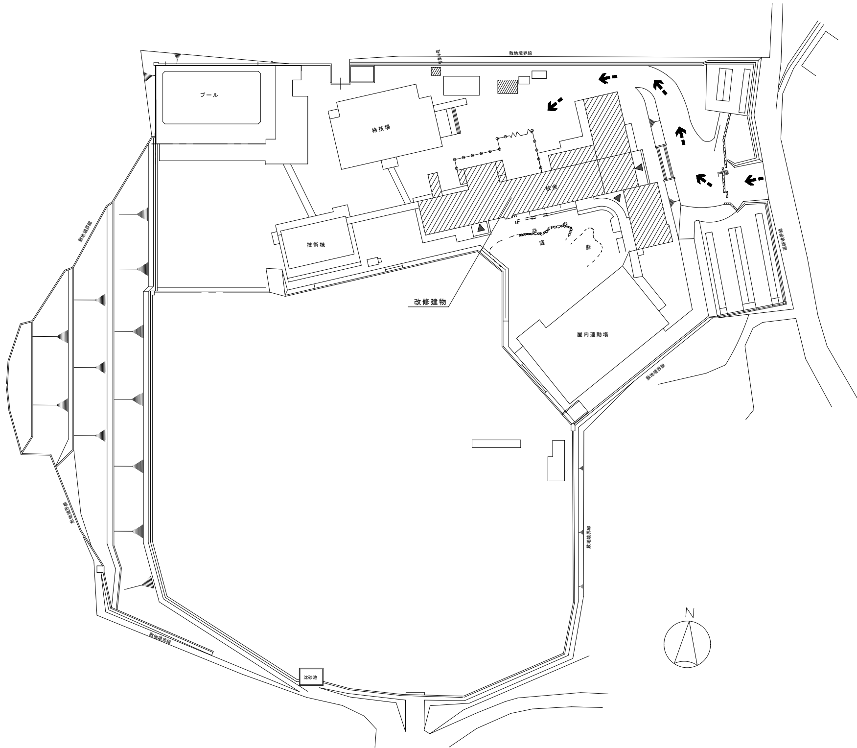
配置図 S=1:500
