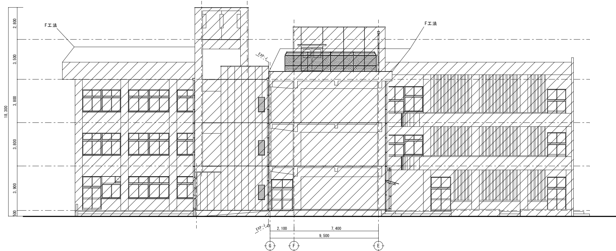
西面立面図 S=1:100
