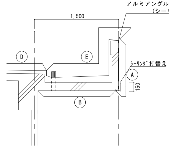
大庇部詳細図 S=1/20
