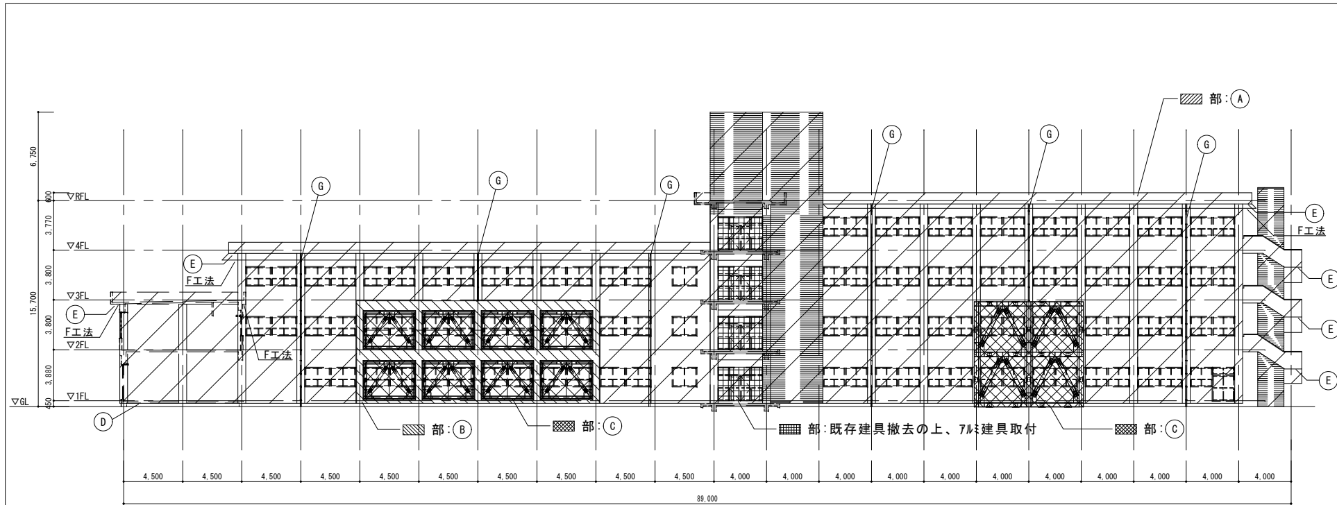
北側立面図 S=1/200
