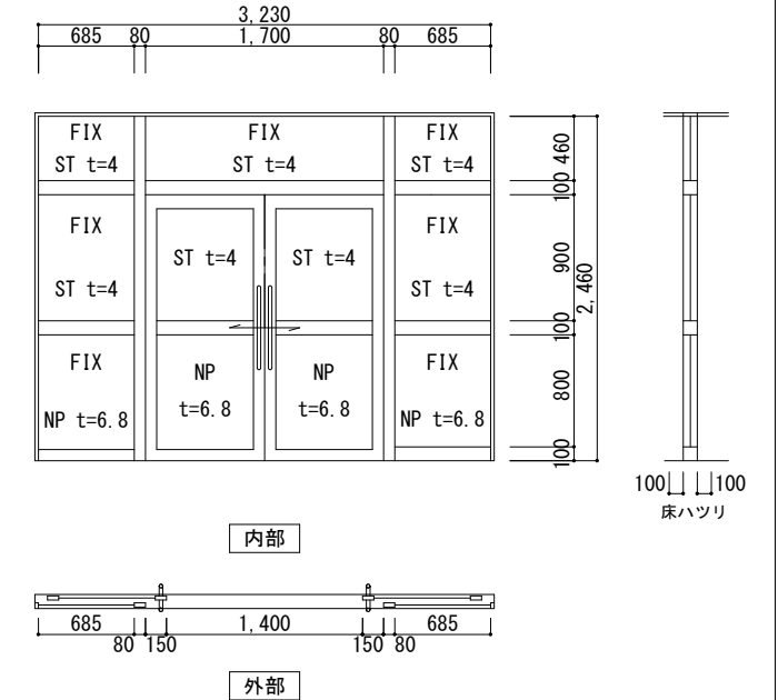
新規建具表 S=1/30
