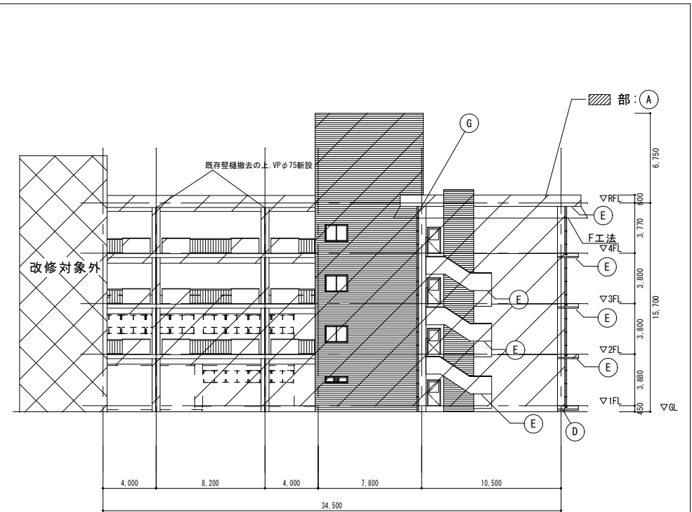
西側立面図 S=1/200
