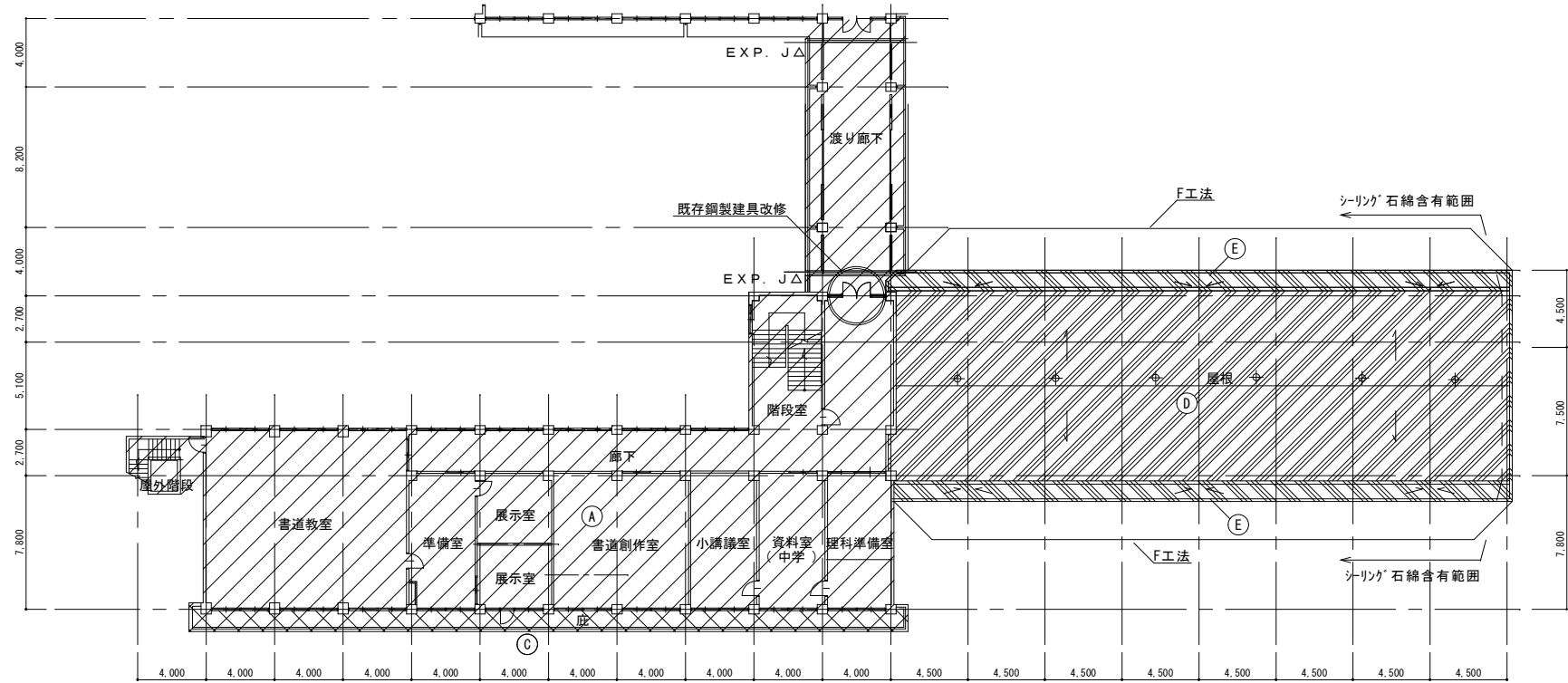
4階平面図 S=1/200
