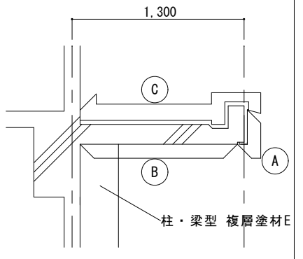
庇詳細図 S=1/20
