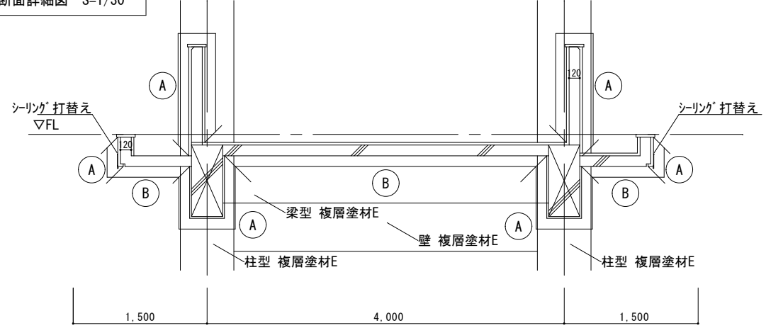
渡り廊下 2・3・4階断面詳細図 S=1/30
