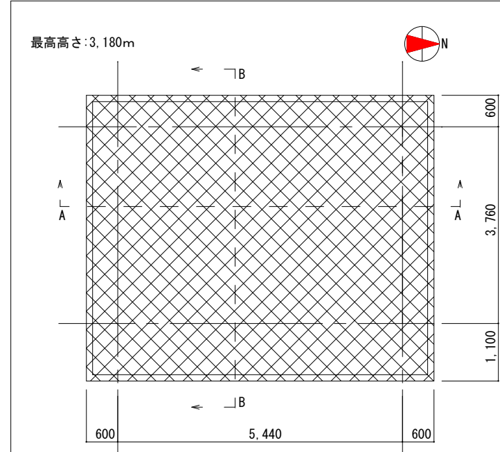
シャワー棟屋根伏図 S=1/100
