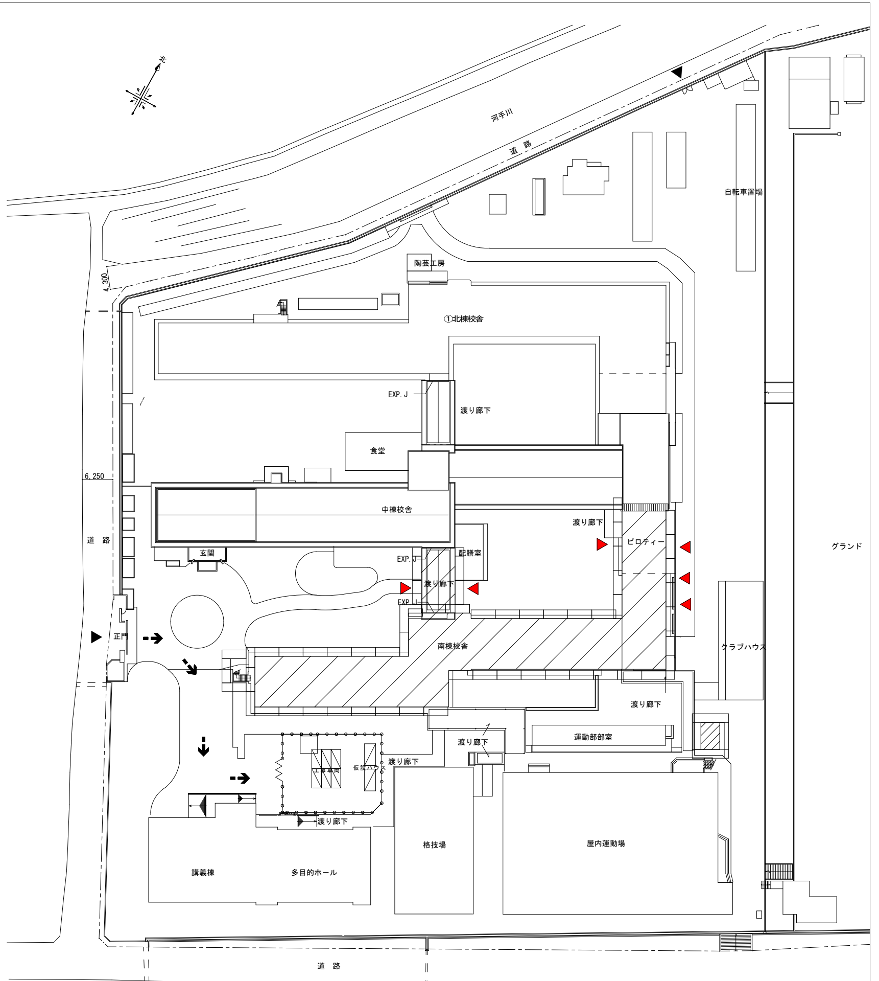
配置図 S=1/400
