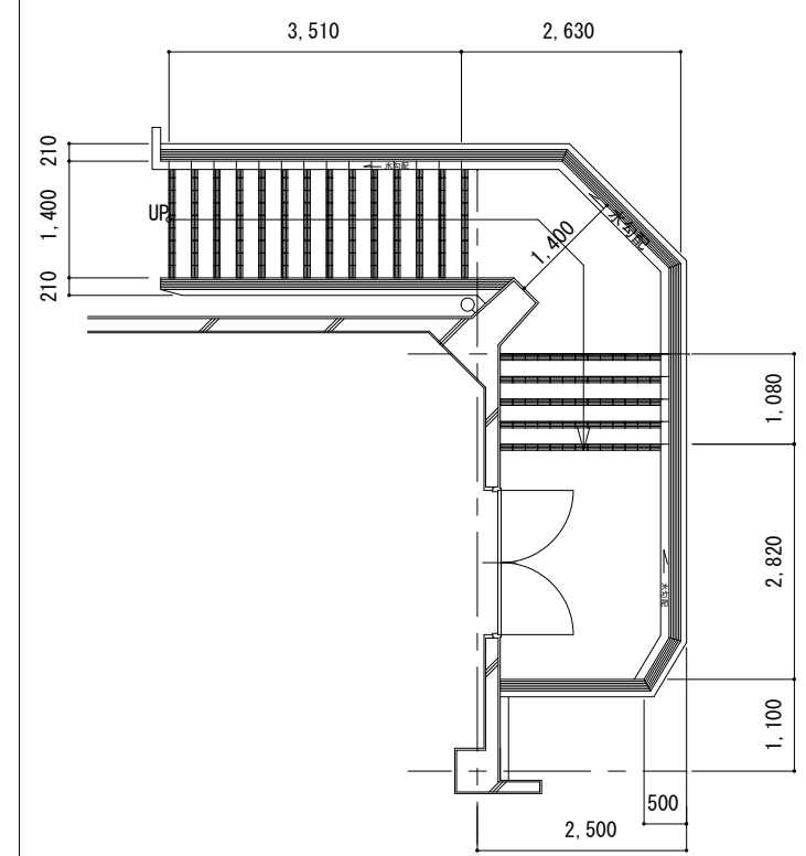
屋内運動場 屋外階段 平面図・断面図 S=1/50
