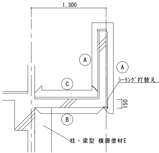
バルコニー詳細図 S=1/20
