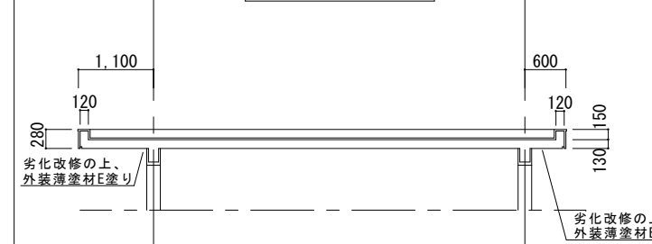
B-B断面図 S=1/50
