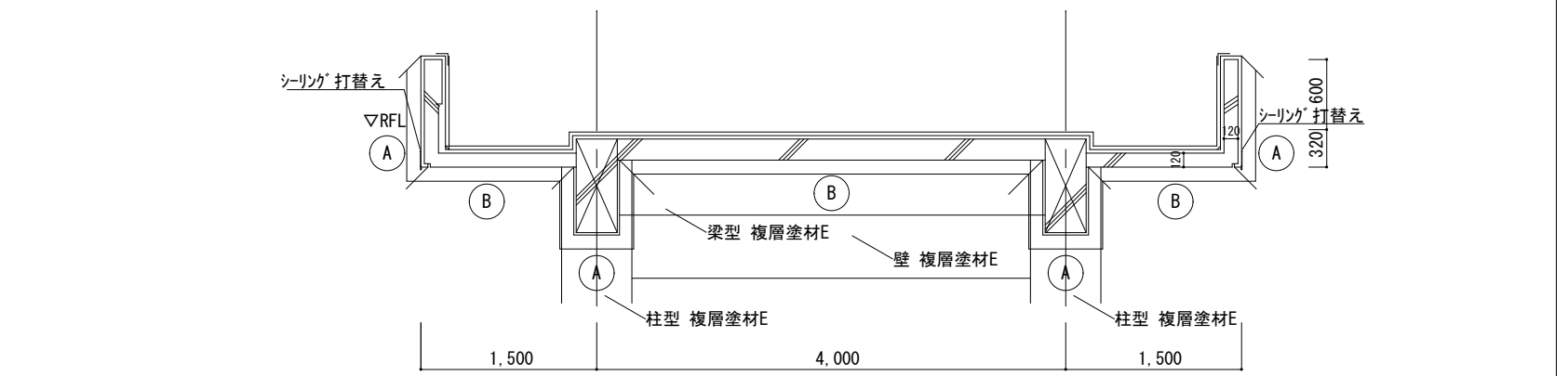
渡り廊下 R階断面詳細図 S=1/30
