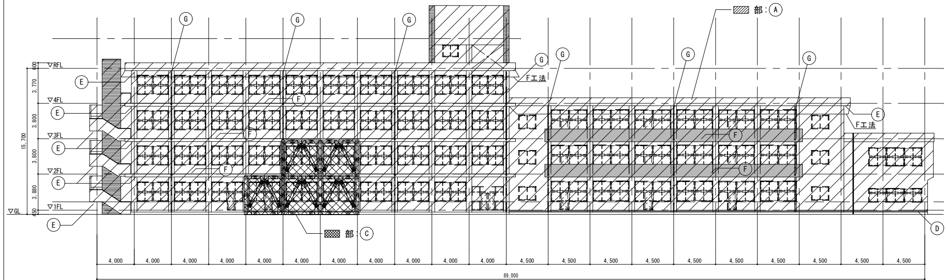
南側立面図 S=1/200
