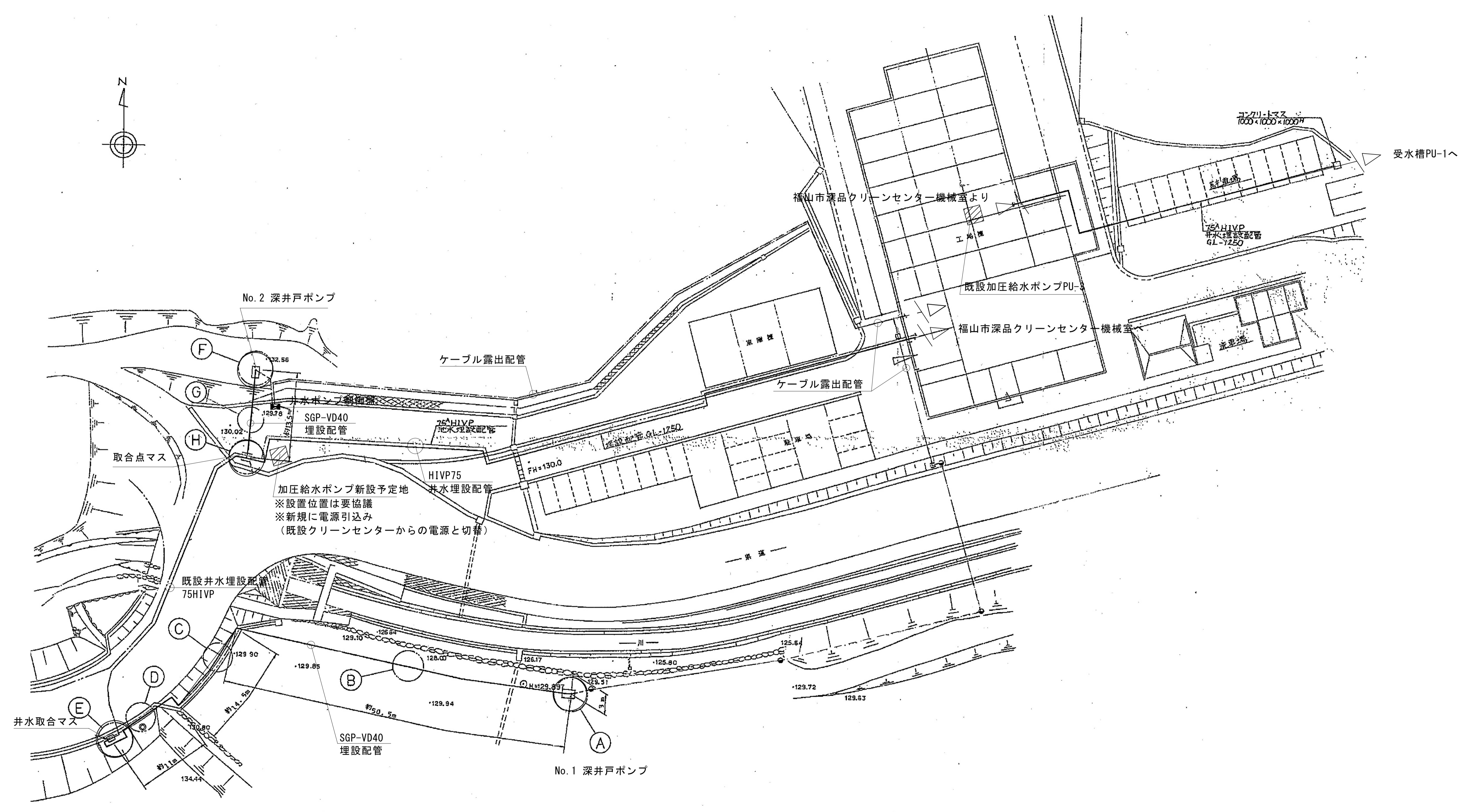
深品クリーンセンター 屋外配管図 No Scale
