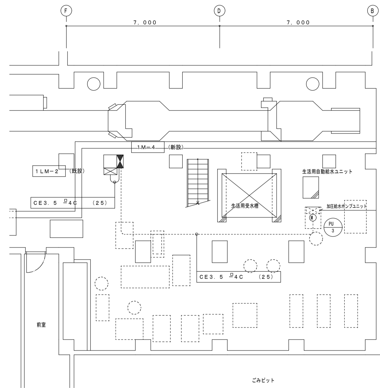
深品クリーンセンター 1階平面図 1/100
