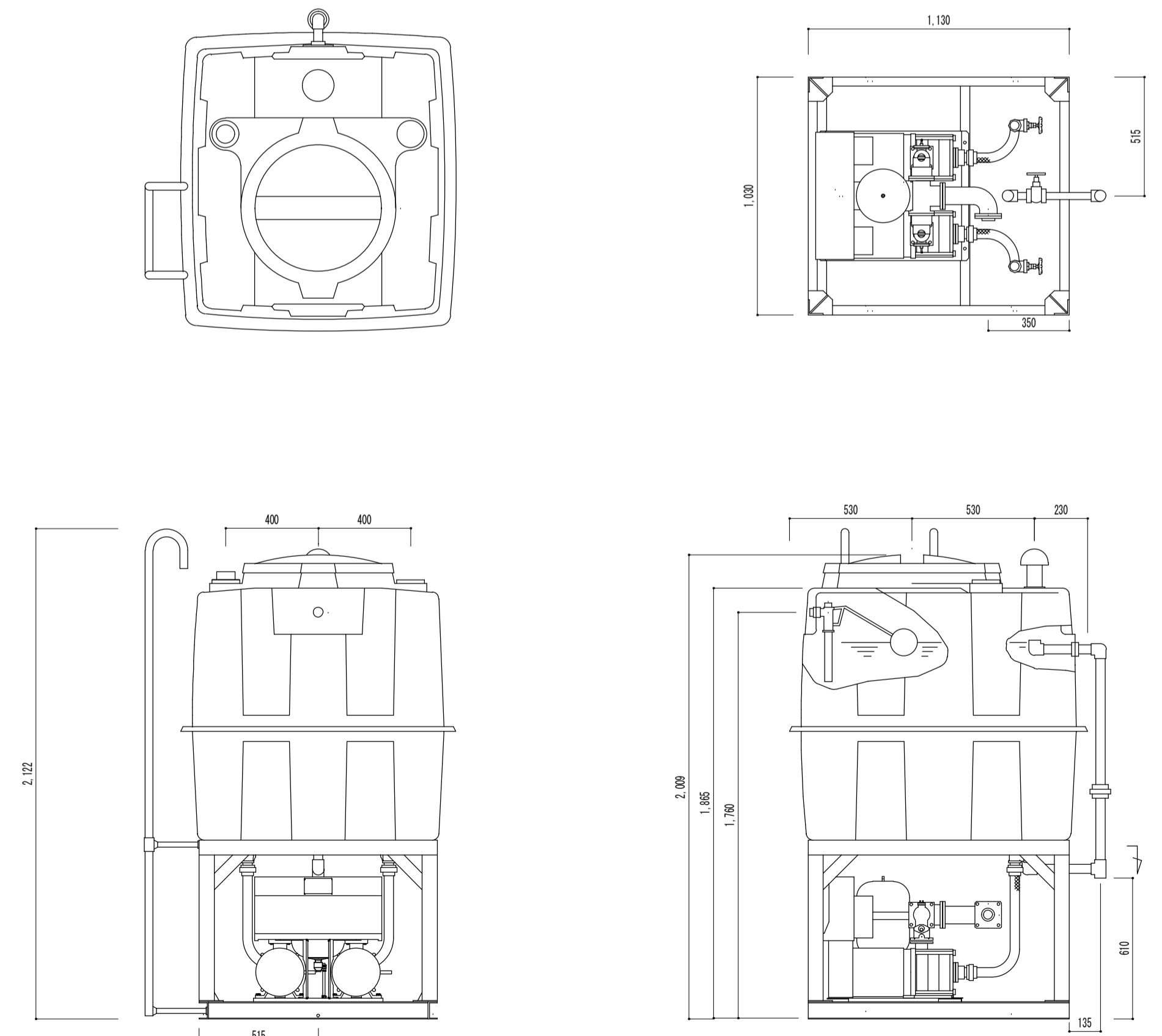
PU 2 受水槽付加圧給水ポンプ（二次側） 参考姿図 1 / 20
