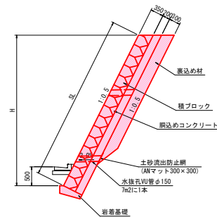
練積ブロック擁壁 S=1:50
