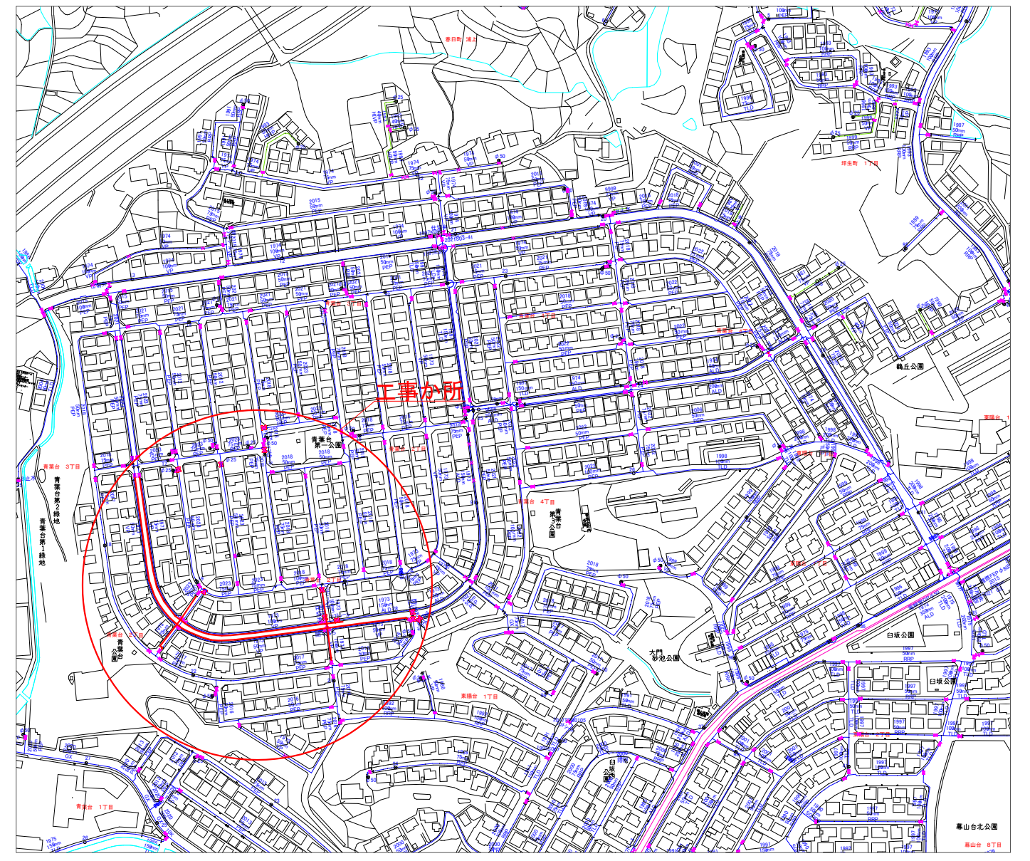
配管図 S=1/2500 *
