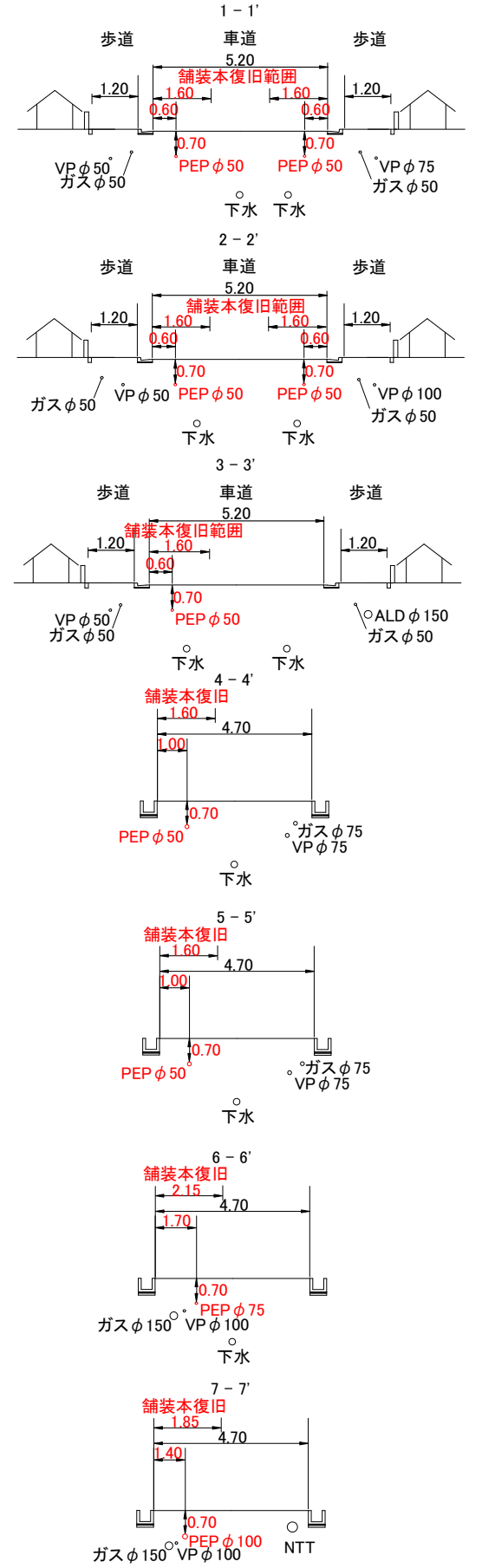
横断面図 S=1/100
