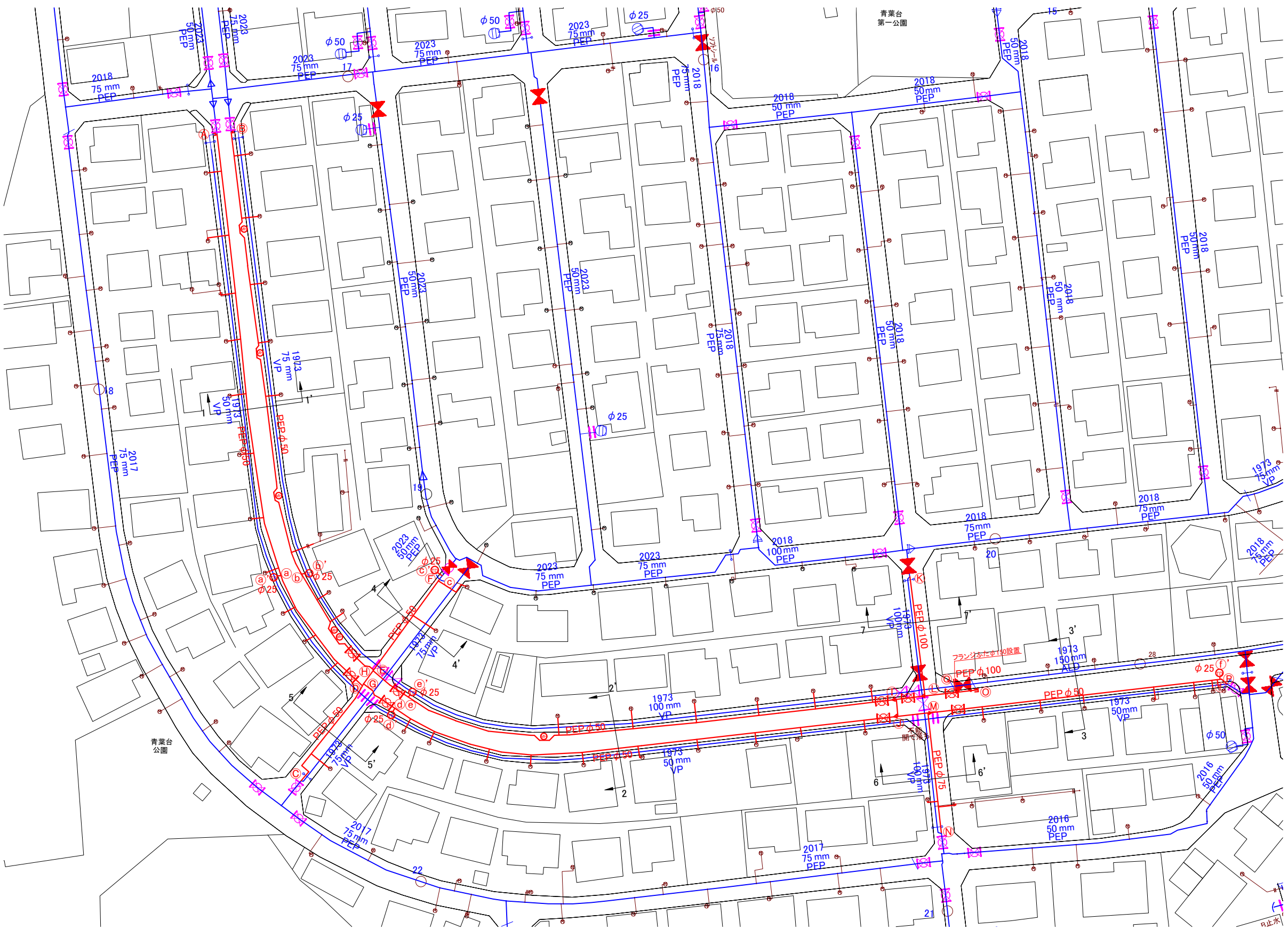
平面図 S=1/500
