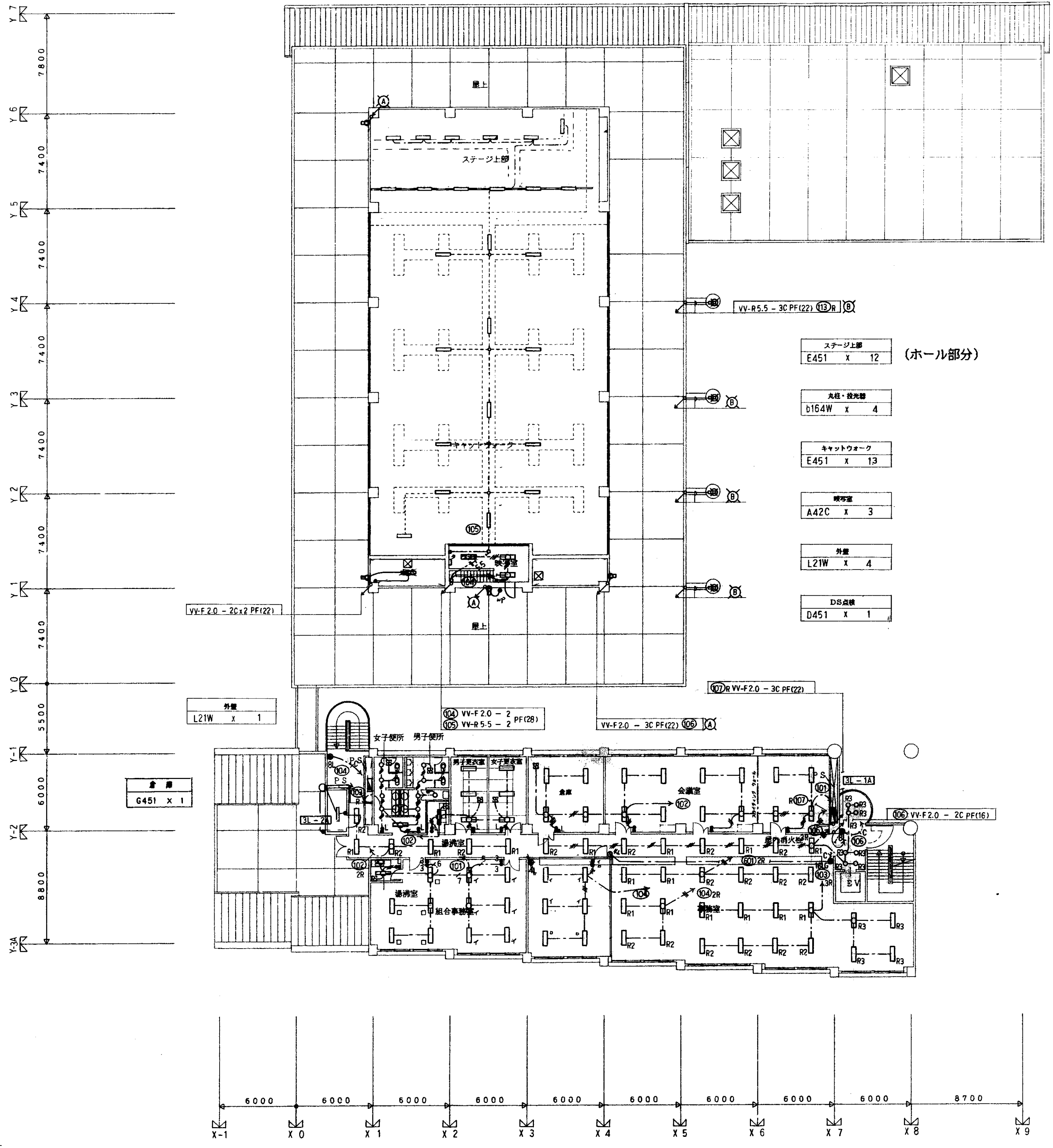
3階平面図 S=1/200
