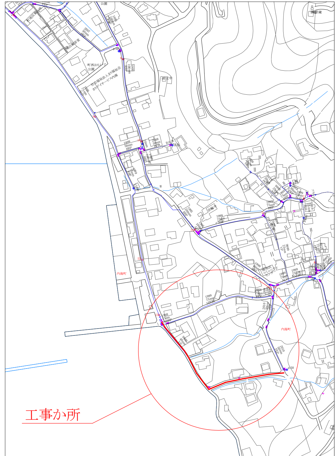
配管図 S=1/2500
