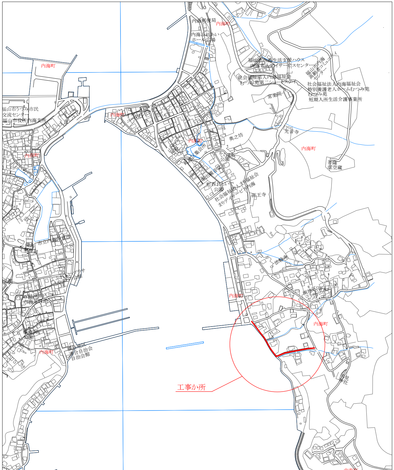
位置図 S=1/5000
