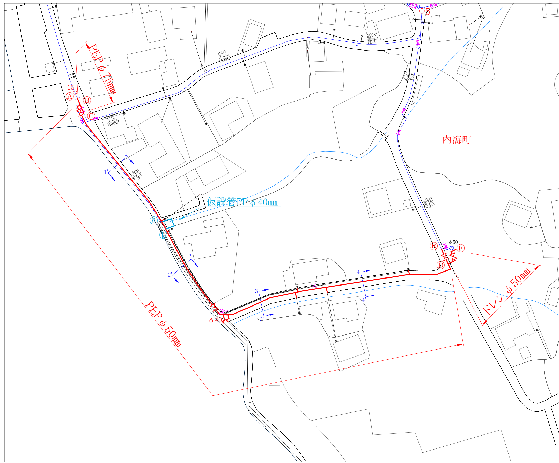
平面図 S=1/500
