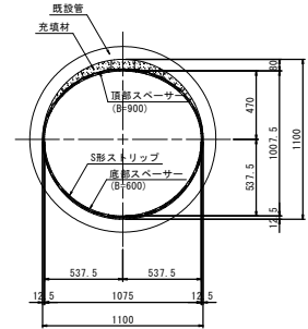
更生管断面図 (参考図面)
