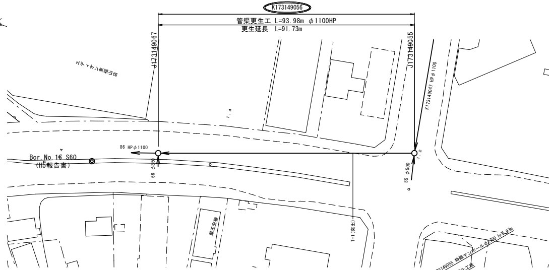
平面図 S=1:500
