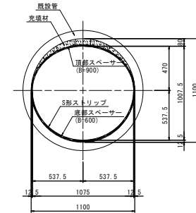
更生管断面図 (参考図面)
