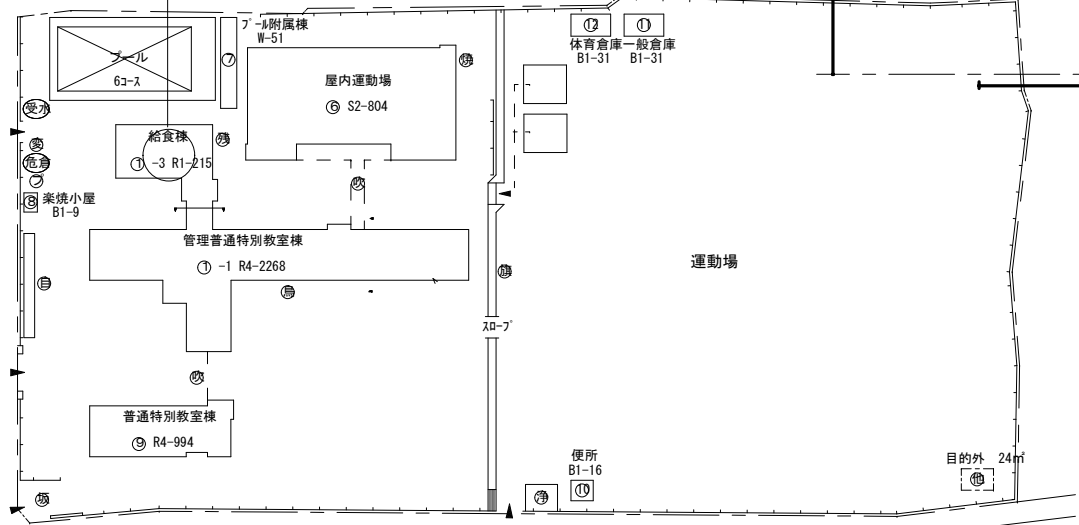
配置図 S = 1 / 1000
