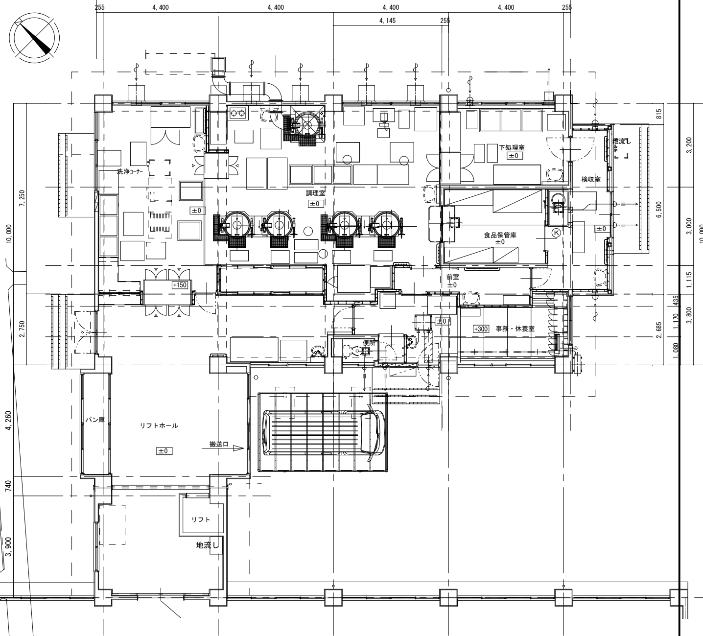
平面図 S = 1 / 100
