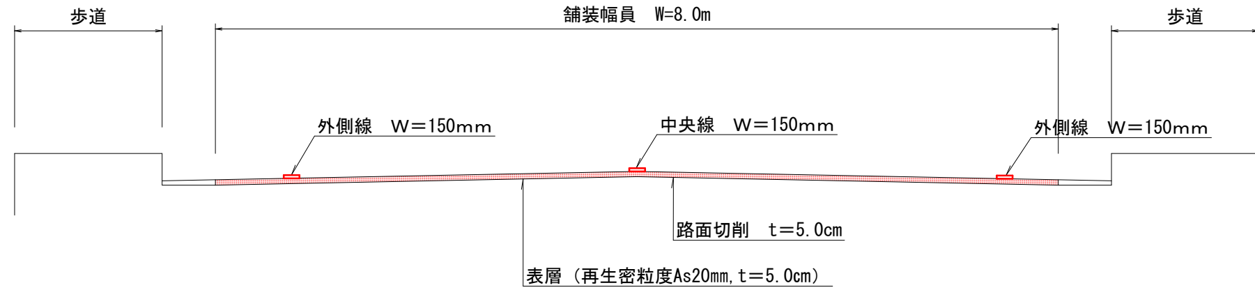
横断図 S=1 : 50
