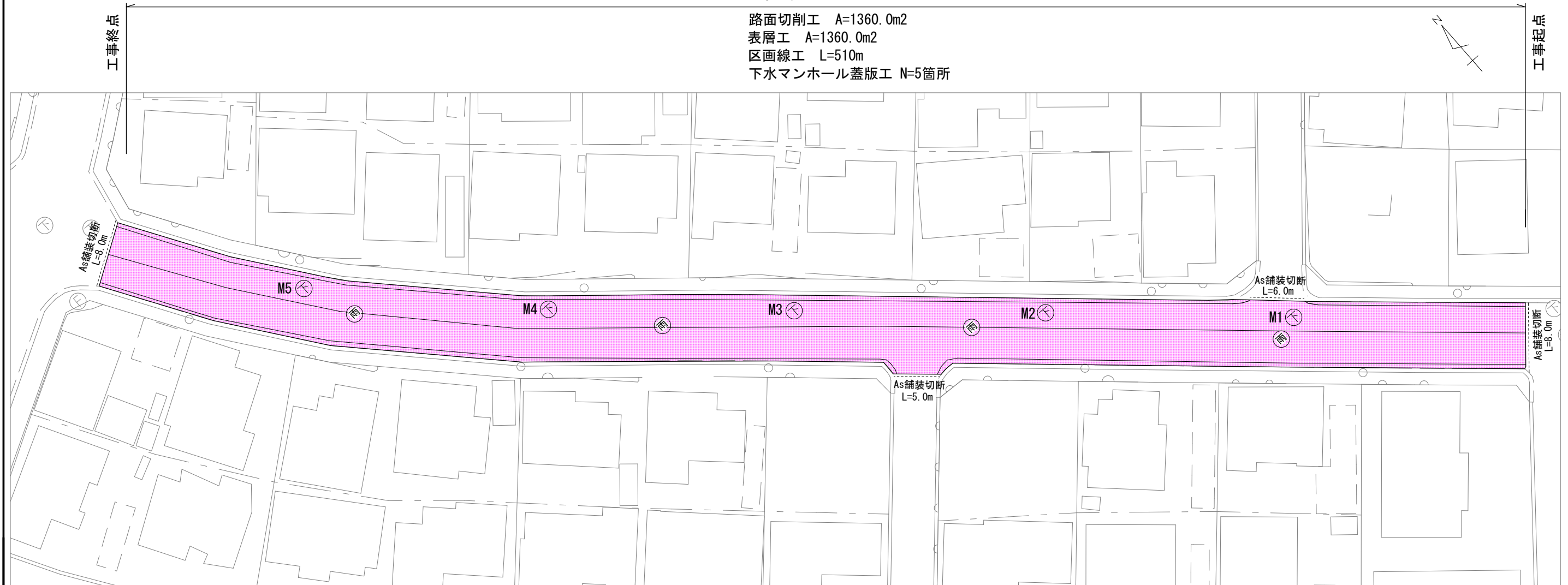
平面図 S=1 : 500
