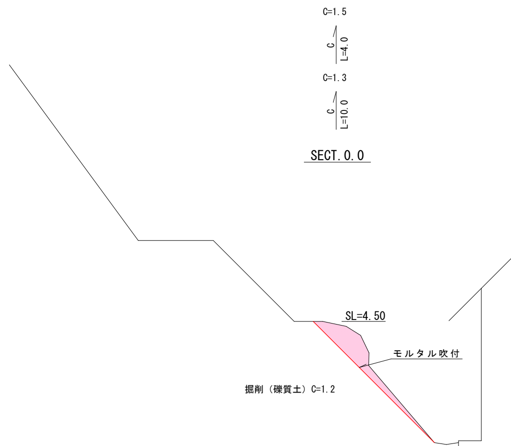
標準横断図 S=1:100
