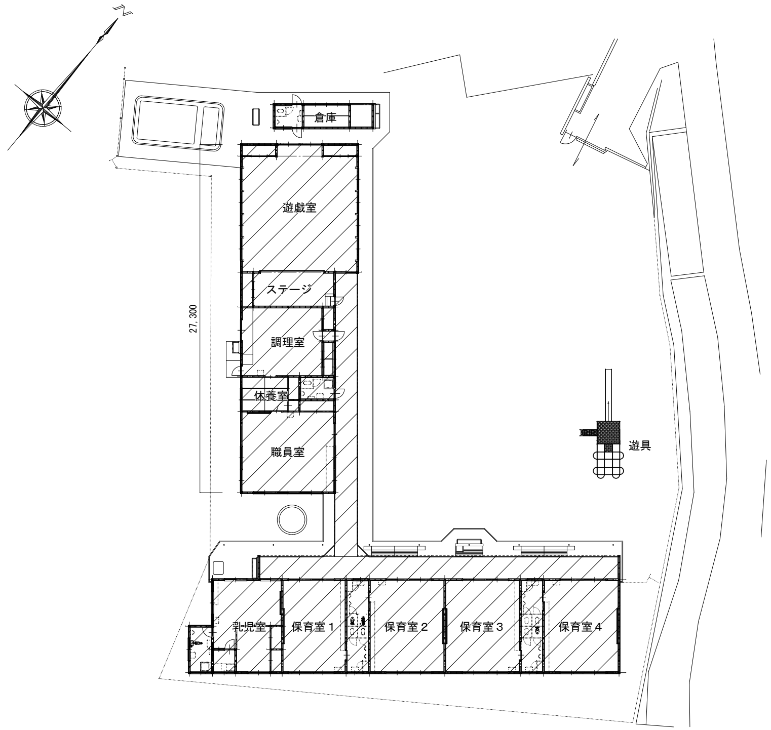
配置図 S=1/300
