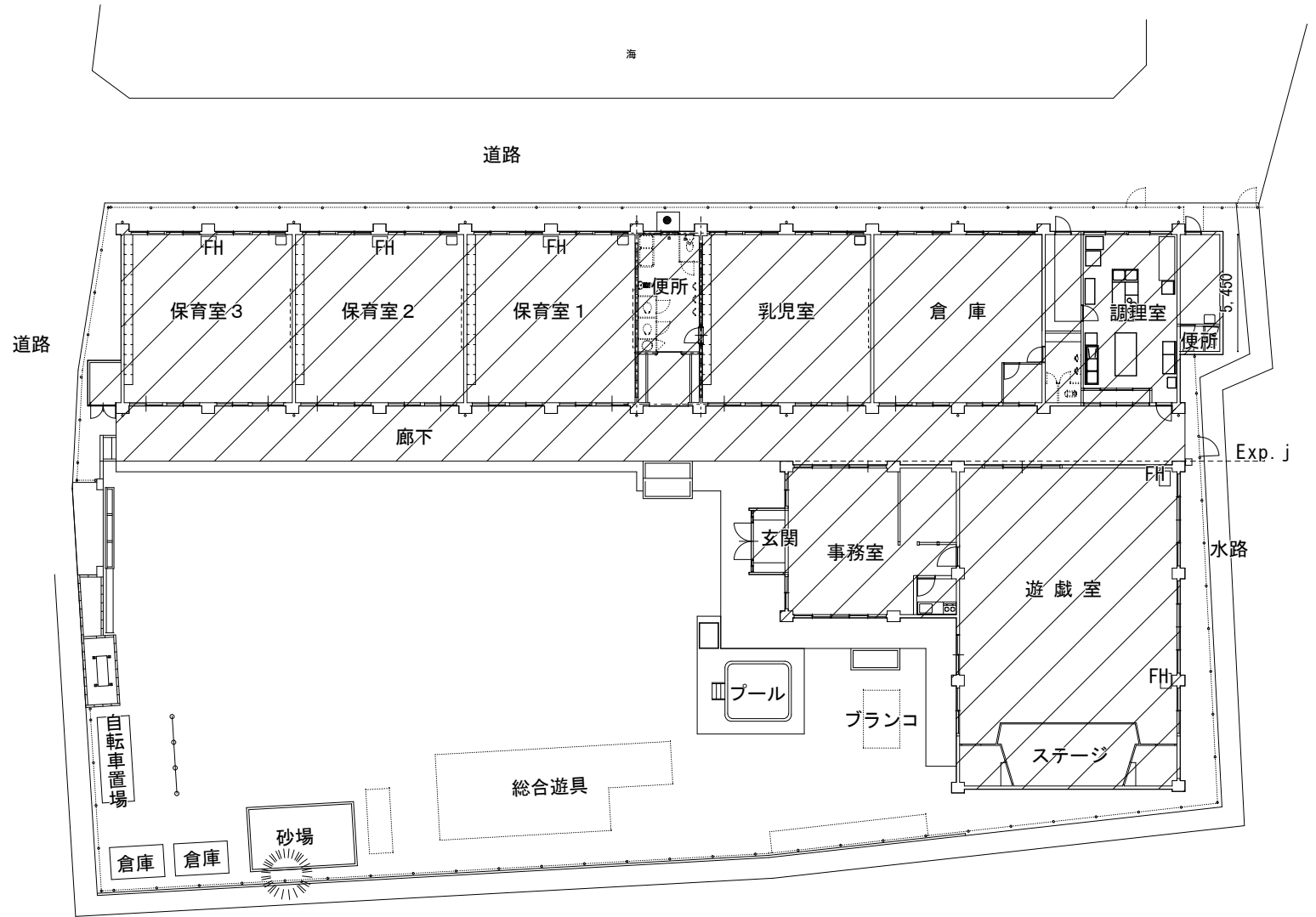
配置図 S=1/300
