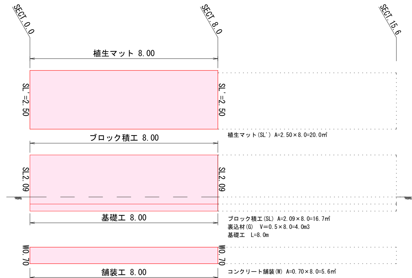
展開図 S=1/100
