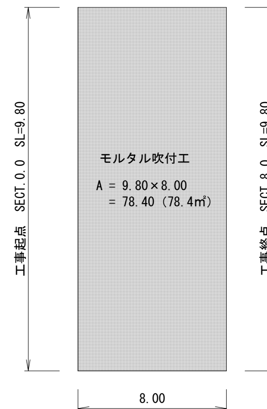
モルタル吹付工 展開図
