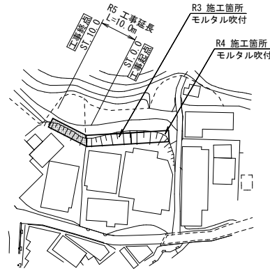
平面図 S=1:1000
