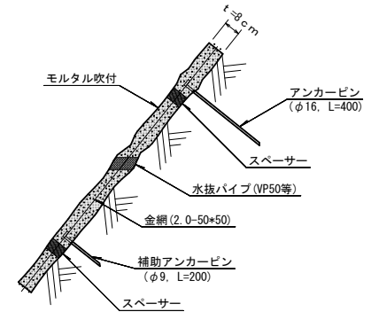
構造図(モルタル吹付) S=1:20
