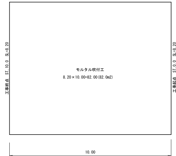
展開図(モルタル吹付) S=1:100
