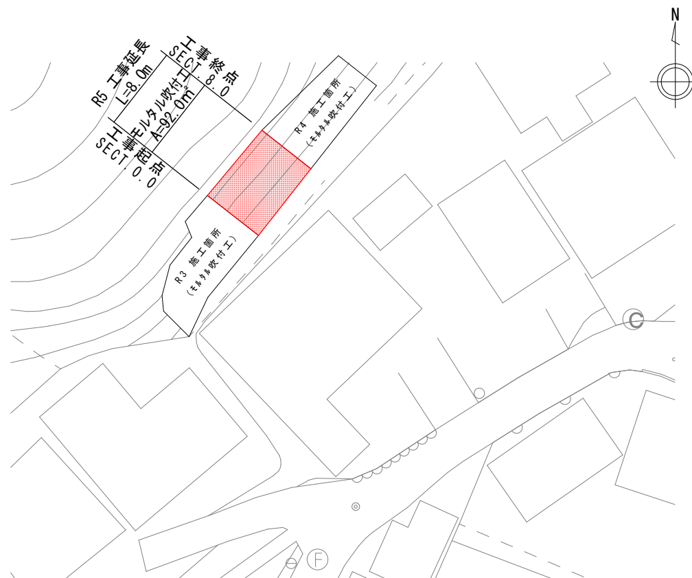
平面図 S=1/500
