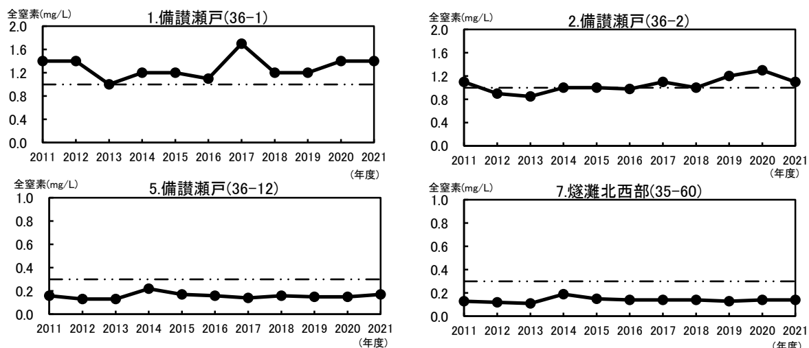
全窒素濃度経年変化（----- は環境基準）
