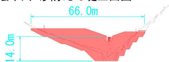
陰平川 砂防えん堤正面図
