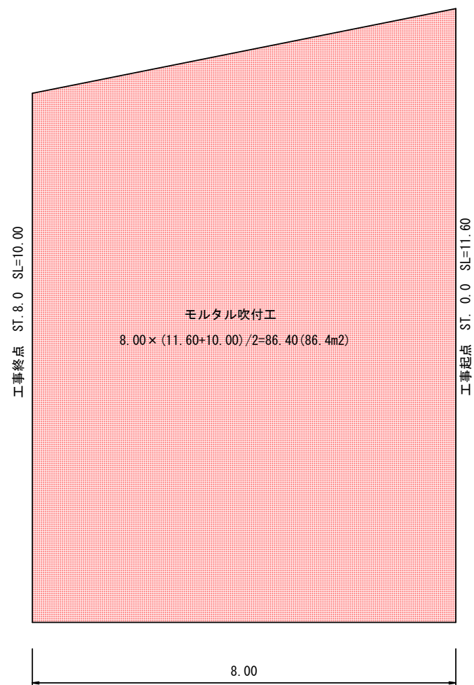
モルタル吹付工 展開図
