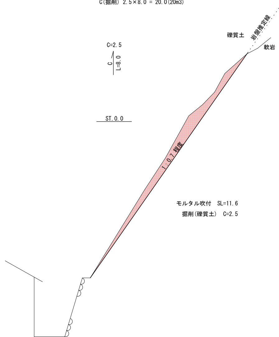
標準横断面図 S=1/100
