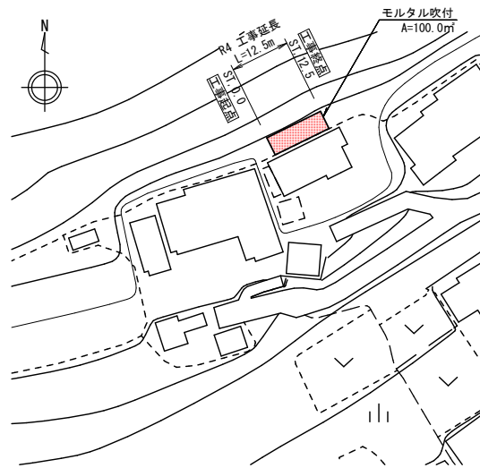
平面図 S=1:1000
