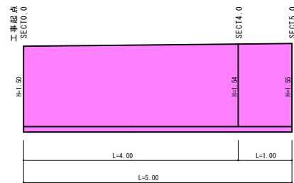
2号重力式擁壁
