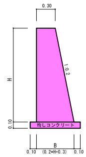
2号重力式擁壁
