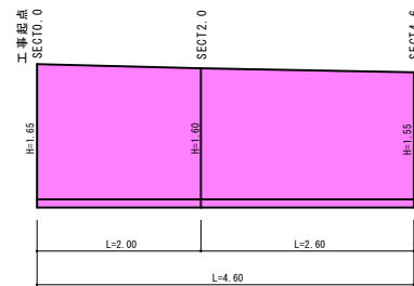
1号重力式擁壁
