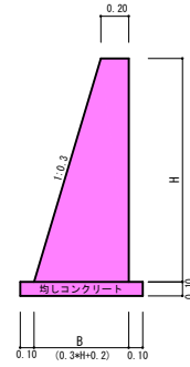
1号重力式擁壁
