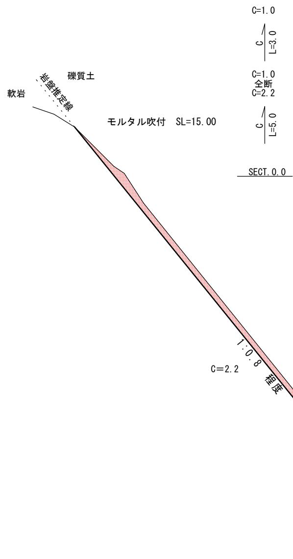
標準横断面図 S=1/100
