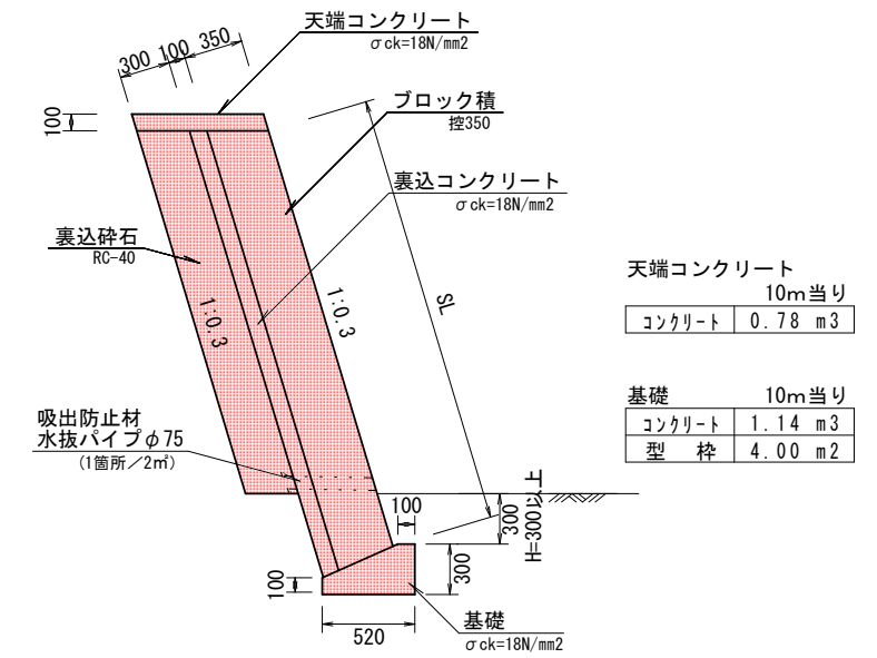
構造図 (ブロック積) S=1:50
