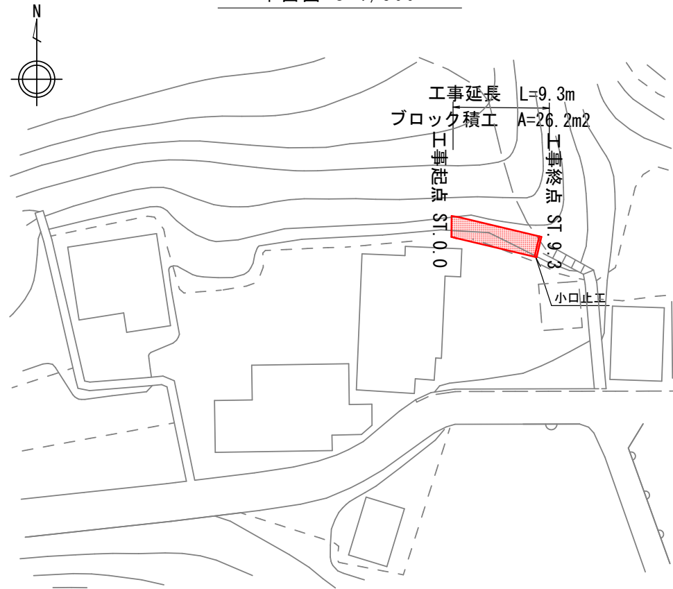
平面図 S=1/500
