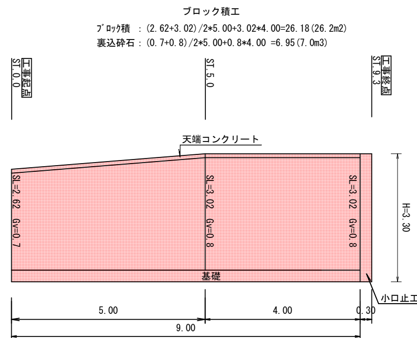
展開図 (ブロック積) S=1:100
