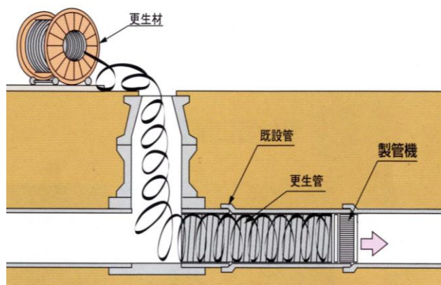
【下水道管渠耐震化工事イメージ】
