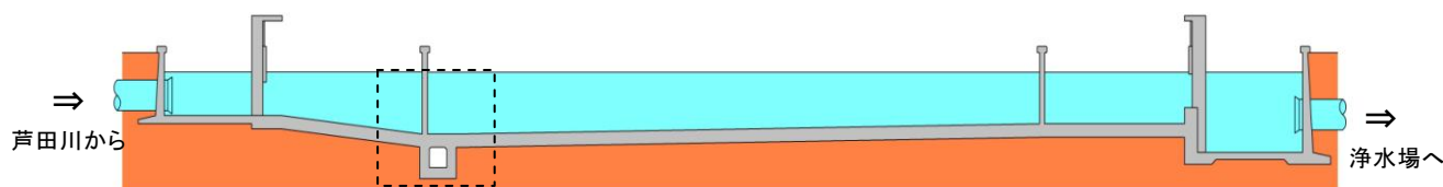
【沈砂池断面図】
