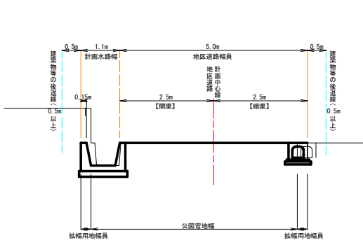
標準断面図
