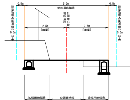
標準断面図
